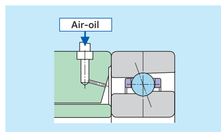
Fig. 9.27 HSF type
