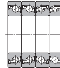
When two rows bear axial load (DTBT)
