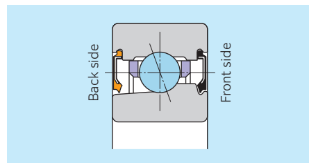
Fig. 9.43 BNS LLB type
