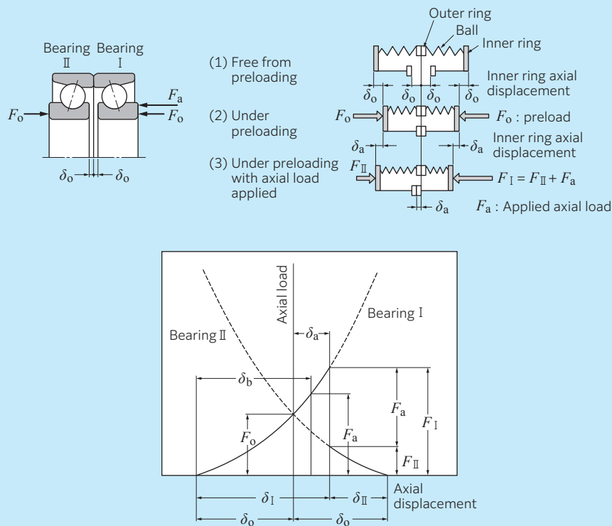
Fig. 2.11 Preload diagram
